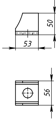
Поз.4 (Ушко)
