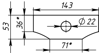
Поз.4 (Ушко) развертка
