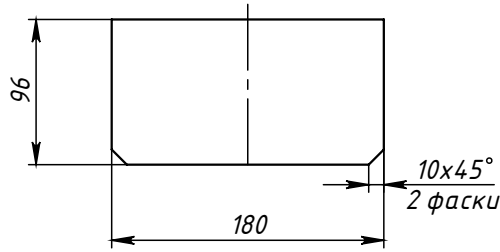
Поз.2 (Ребро)
