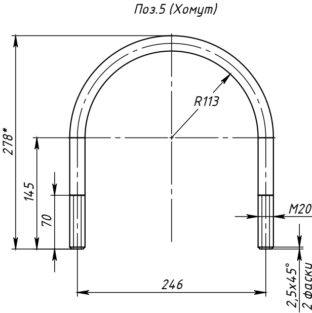
Поз.5 (Хомут)
